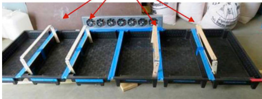
Расми 4. Тарафи чап: Чор қолиби нигоҳдоранда дар рӯи табақчо ҷой дода шудаанд. Тарафи рост: як охири қолиби нигоҳдоранда, ки бо изолента маҳкам карда шудааст.
