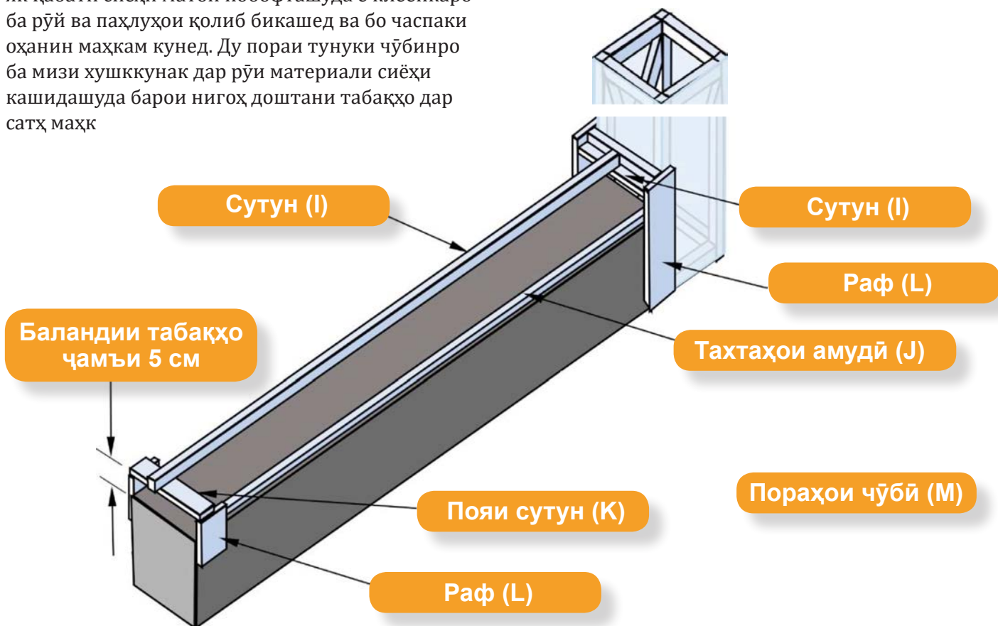
Расми 4. Ангораи дудкаш, ки ба мизи хушккунак пайваст карда шудааст
