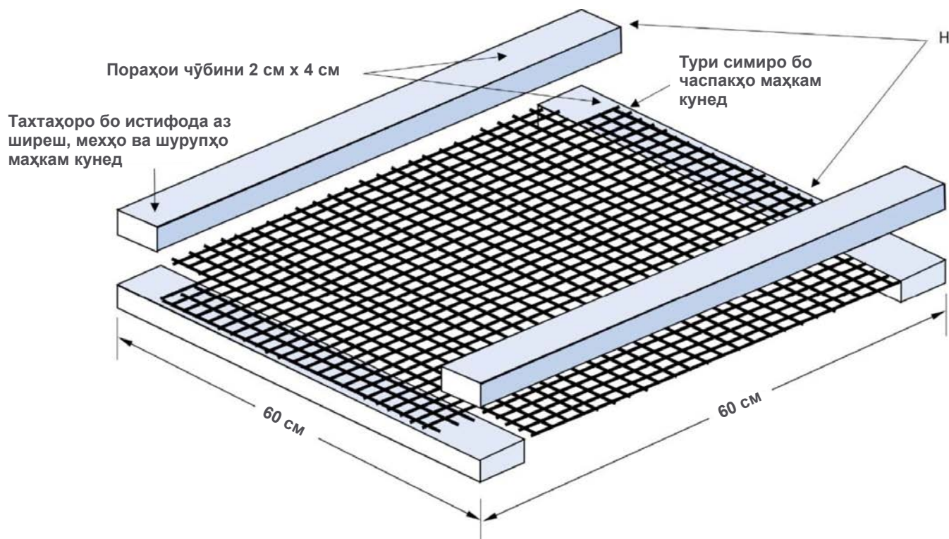
Расми 5. Намои васеи табақи хушккунак
