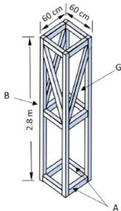
Расми 3. Қолиби чӯбӣ барои дудкаш
